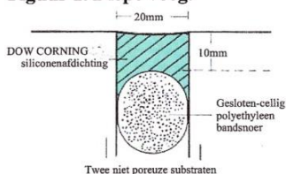
Figuur 2: Ondiepe voeg.
